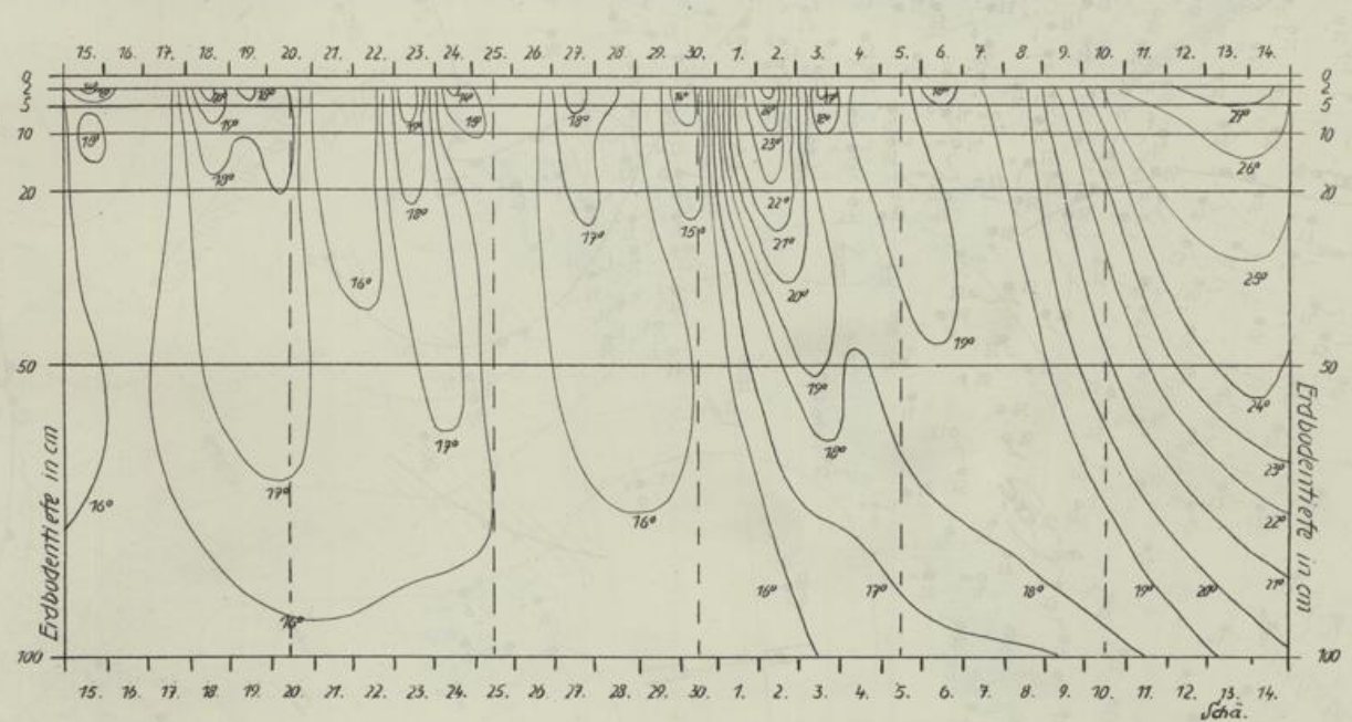
Verlauf der Erdbodentemperaturen in Potsdam in der Zeit vom 15. Juni bis 14. Juli 1956
