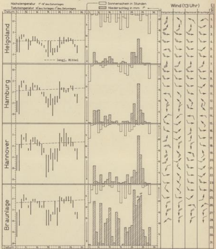
Etwas zu -Deutsche Sicht und wäuliche Orkne- Witterungsverlauf im Februar 1970 von Mittwoch, den 18. März 1970 Die Darstellung der Temperatur zu P.S. "Föhnwind" bezieht sich auf die Zeit von 11.3. - 16.3.1970
