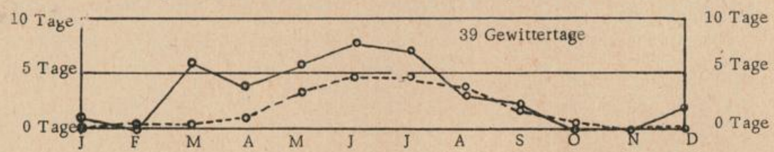
Monatliche Zahl der Gewittertage im Jahre 1966 in Essen (—) im Vergleich zu den langjährigen Mittelwerten (----).
