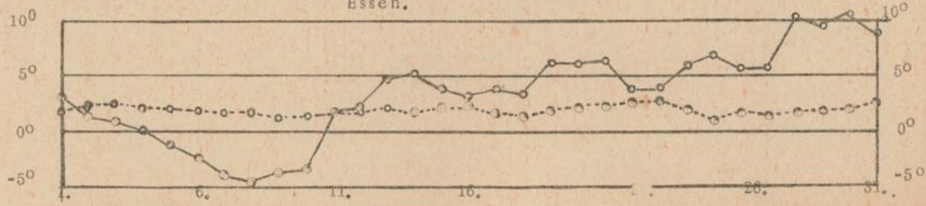
Temperaturverlauf im Januar 1967 (Tagesmittel) im Vergleich zu den langjährigen Mitteltemperaturen des Januar (-----) in Essen.
