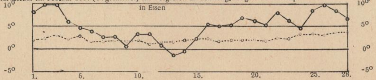
Temperaturverlauf im Februar 1967 (Tagesmittel) im Vergleich zu den langjährigen Mitteltemperaturen des Februar (-----) in Essen
