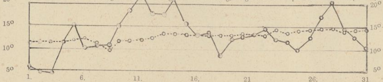
Temperaturverlauf im Mai 1967 (Tagesmittel) im Vergleich zu den langjährigen Mitteltemperaturen des Mai (----) in Essen
