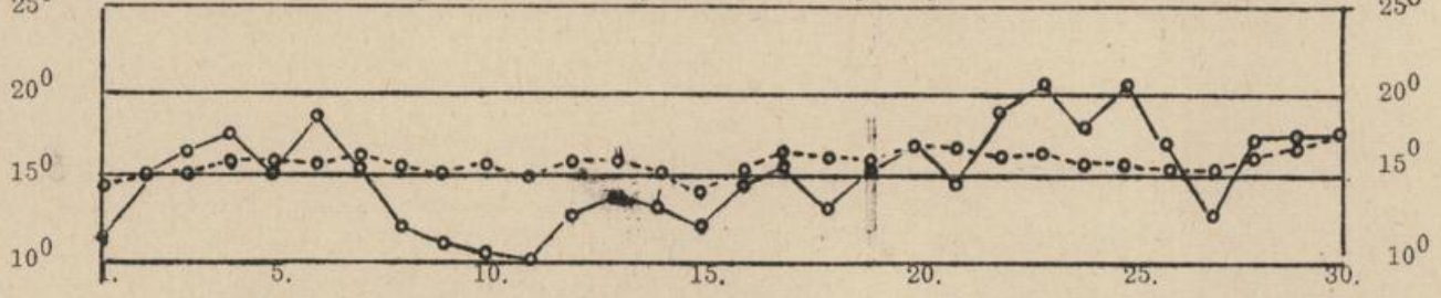
Temperaturverlauf im Juni 1967 (Tagesmittel) im Vergleich zu den langjährigen Mitteltemperaturen (-----) in Essen.
