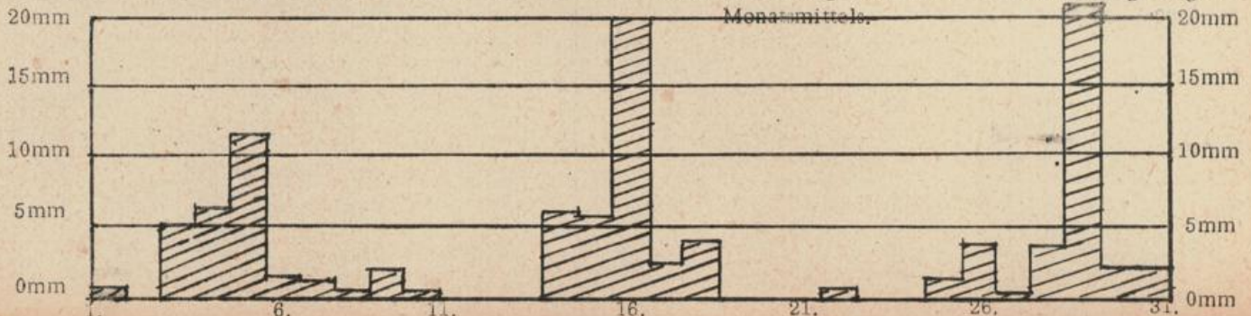
Tägliche Niederschlagsmengen im Oktober 1967 in Essen. Gesamtniederschlag: 99.9 mm = 123,3% des langjährigen Monatsmittels.
