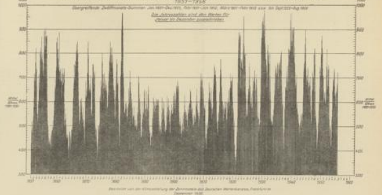
Schwankungen der jährlichen Niederschlagshöhe (mm) in Frankfurt/M. 1857-1956
