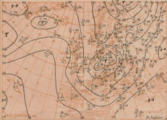
Absolute Topographie 500 mb 3 Uhr (geopot. Dekameter)
