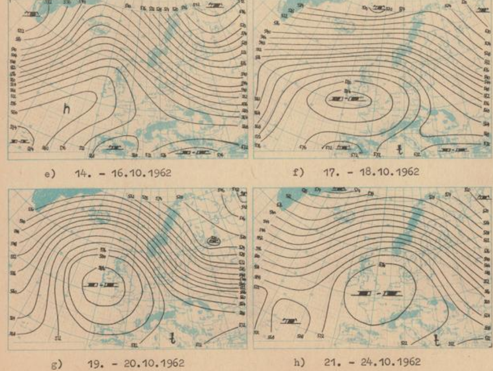
MITTLERE ABSOLUTE TOPOGRAPHIE 500 mbar FÜR FOLGENDE ZEITABSCHNITTE:
