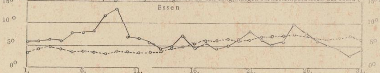
Temperaturverlauf im März 1967 (Tagesmittel) im Vergleich zu den langjährigen Mitteltemperaturen des März (---) in Essen
