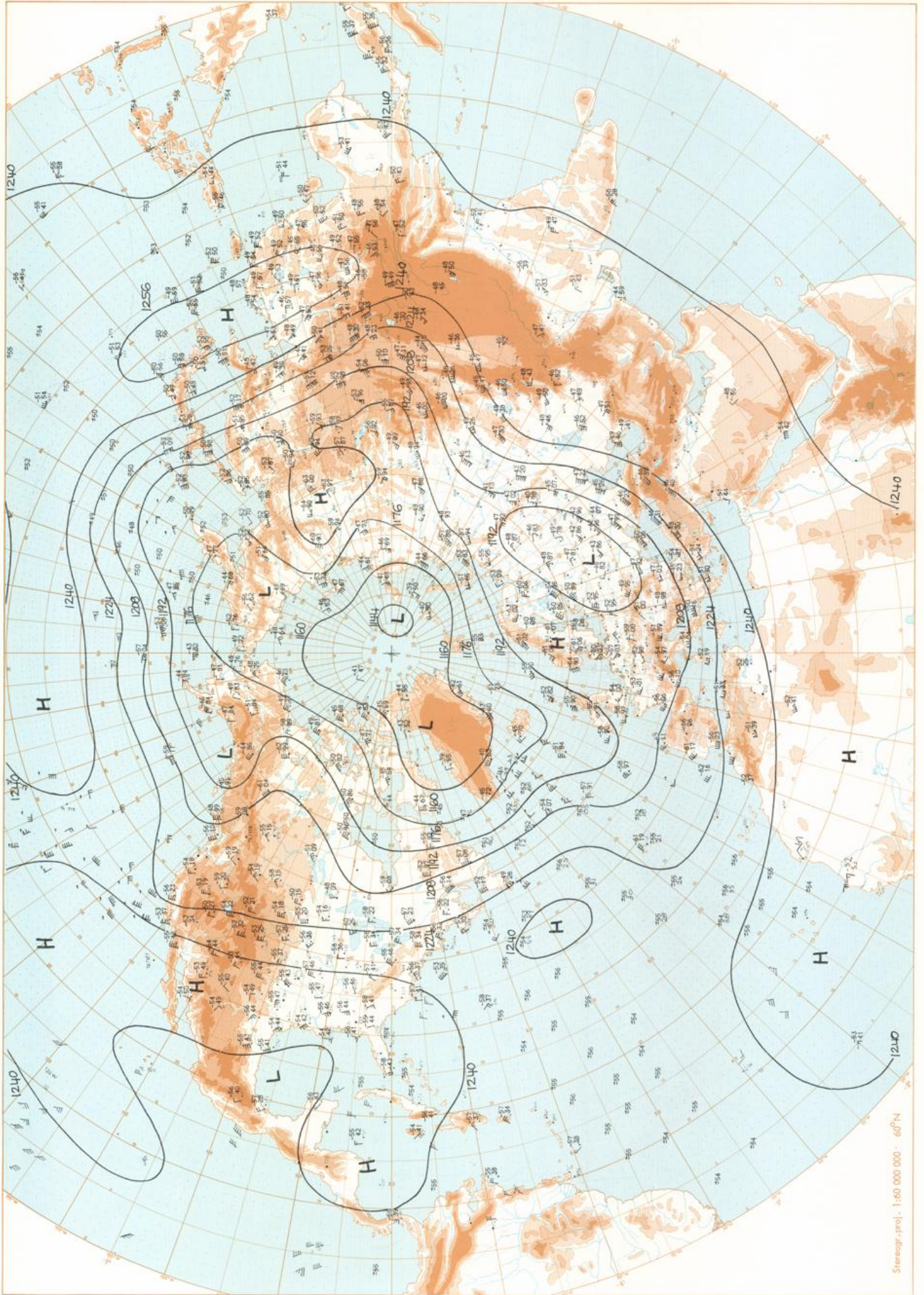
200 mbar 00 GMT
