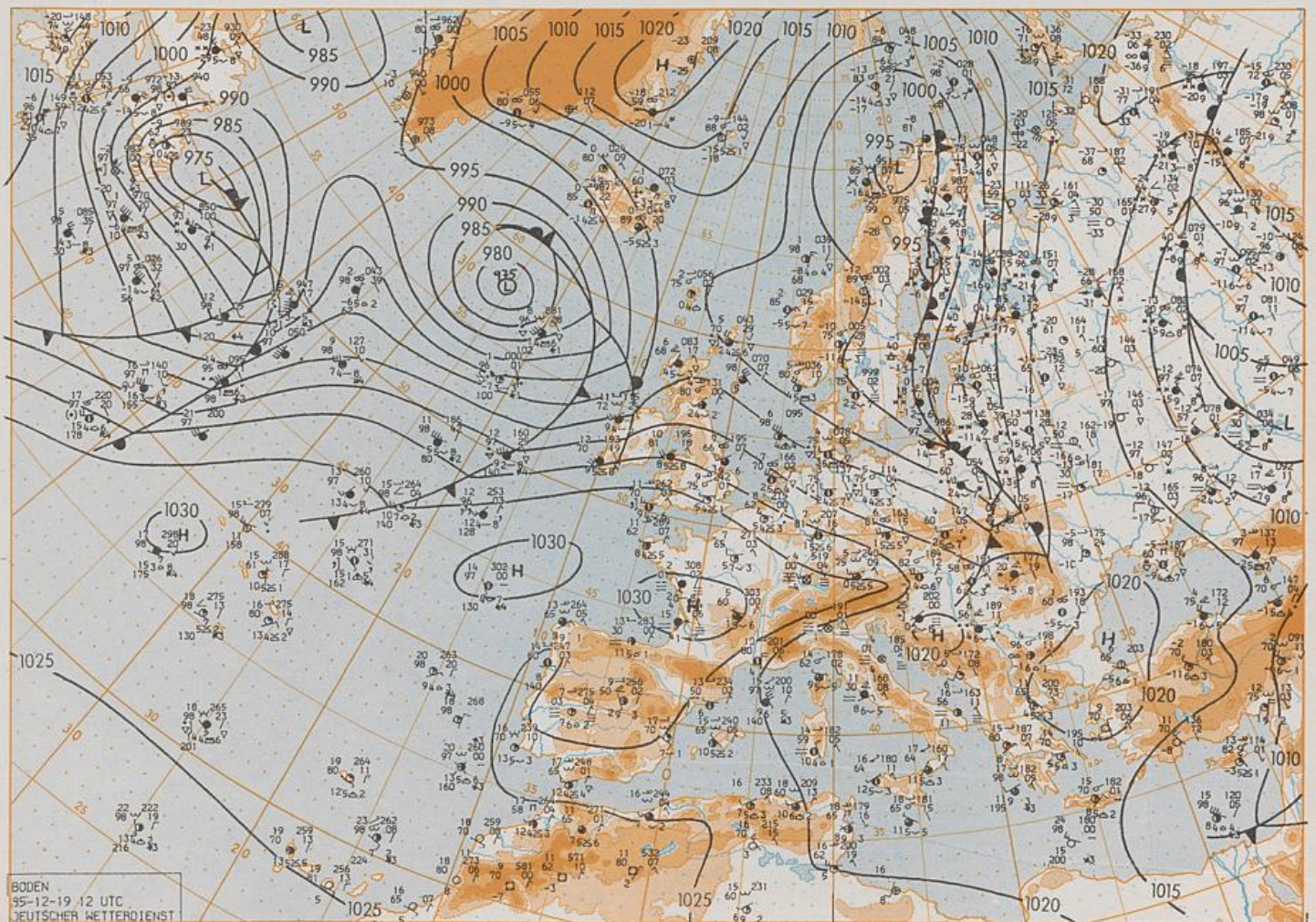
BODEN 95-12-19 12 UTC DEUTSCHER WETTERDIENST Stereogr. proj. 1:30 000 000. 60°N
