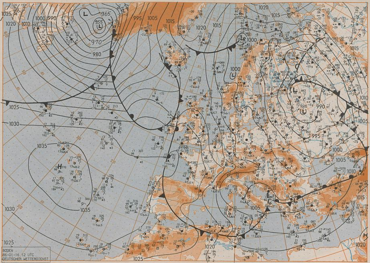
BODEN 86-01-16 / 12 UTC DEUTSCHER WETTERDIENST Stereogr. proj. 1:30 000 000 60°N
