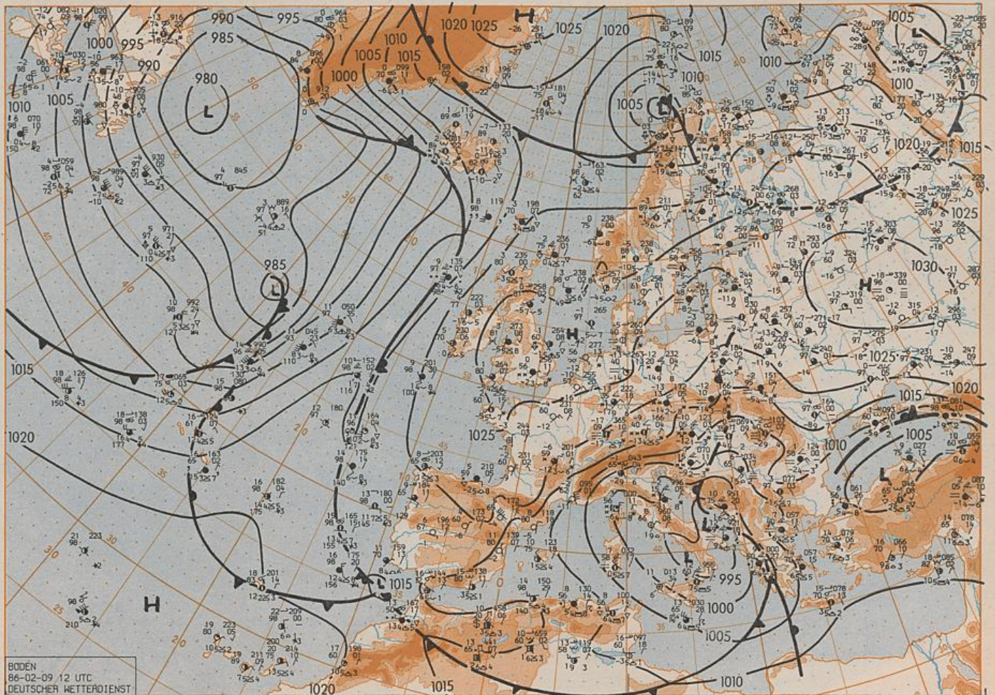
BODEN 86-02-09 12 UTC DEUTSCHER WETTERDIENST Stereogr. proj. 1:30 000 000 60°N
