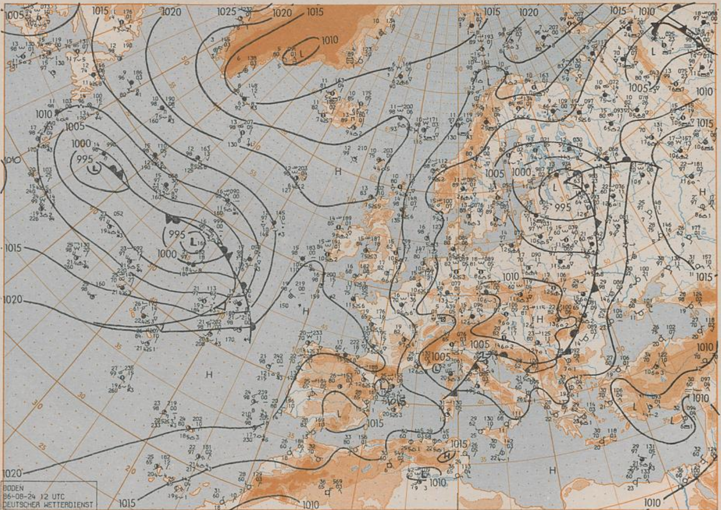
Stereogr.-proj., 1:30 000 000, 60°N
