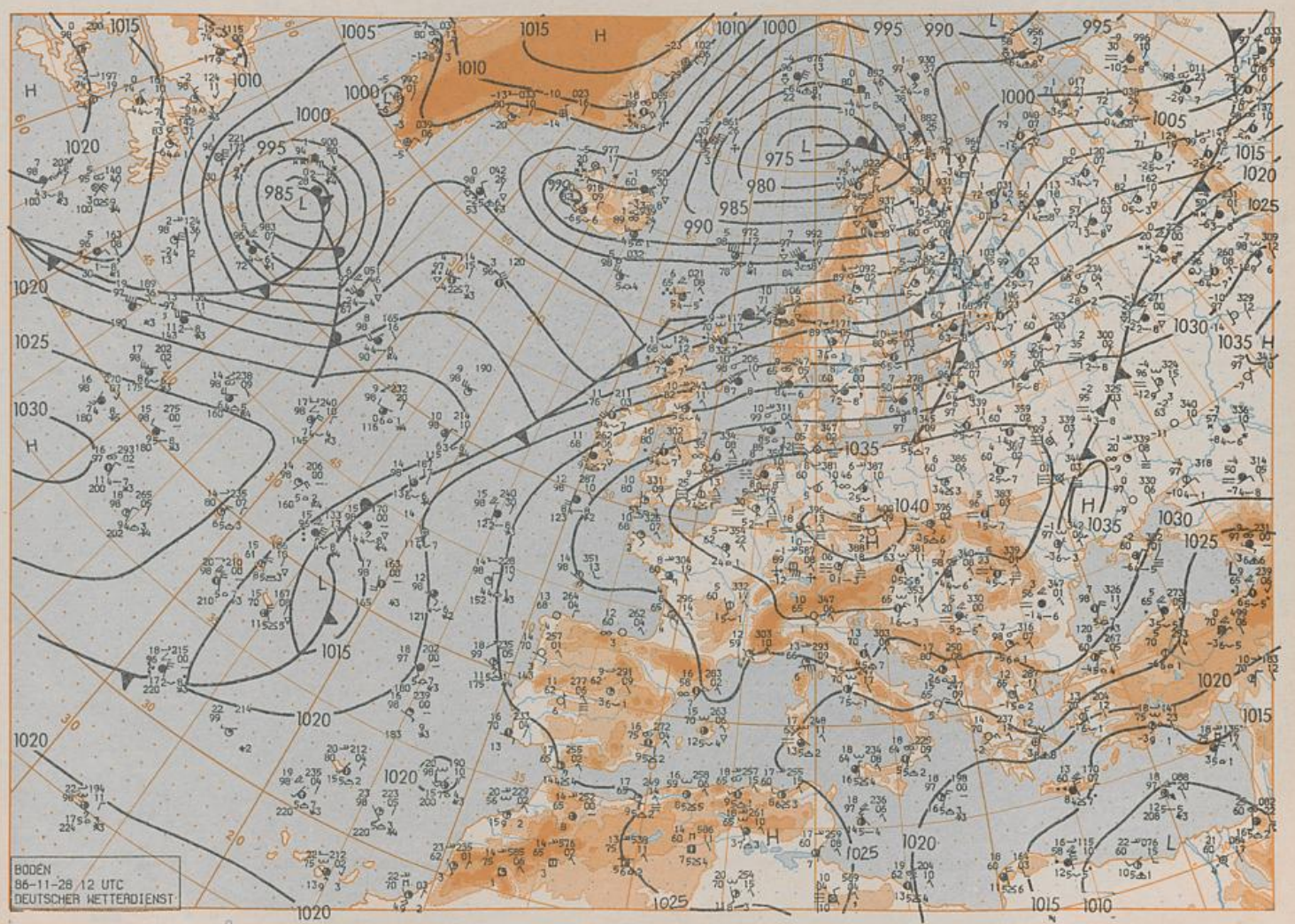
Stereogr. proj., 1:30 000 000 60°N Surface chart 12 UTC
