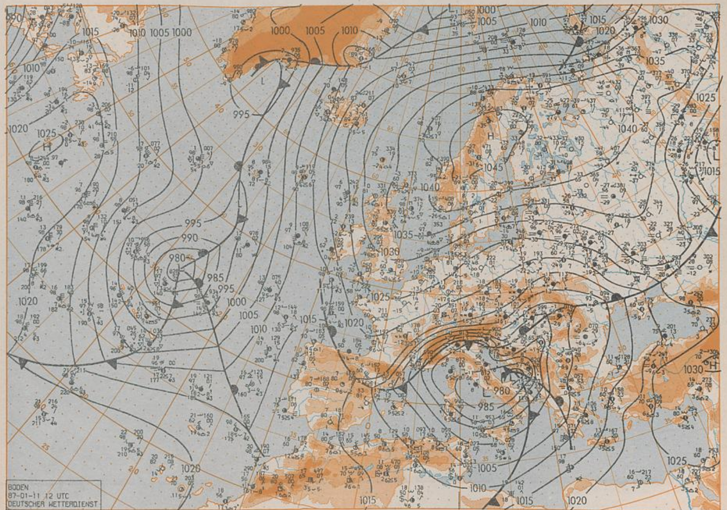
BOEEN 87-01-11 12 UTC DEUTSCHER WETTERDIENST Stereogr. proj. 1:30 000 000 60°N
