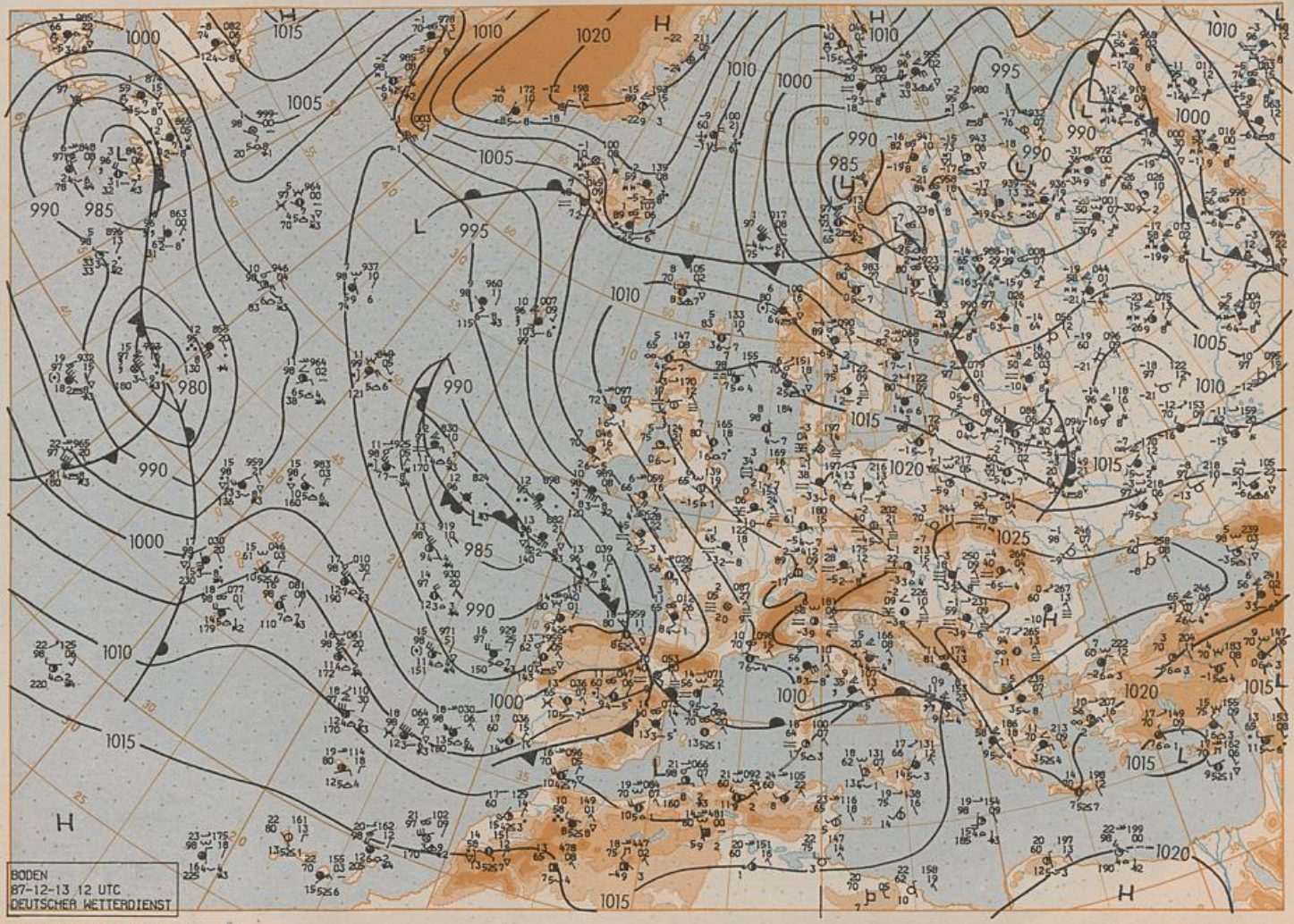
BODEN 87-12-13 12 UTC DEUTSCHER WETTERDIENST Stereogr. proj. 1:30 000 000 60°N Surface chart 12 UTC
