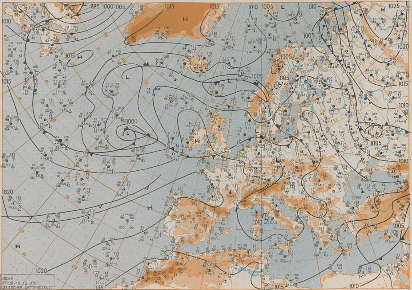
BODEN 87-08-18 12 UTC DEUTSCHER WETTERDIENST Stereoogr. proj. 1:30 000 000 60°N
