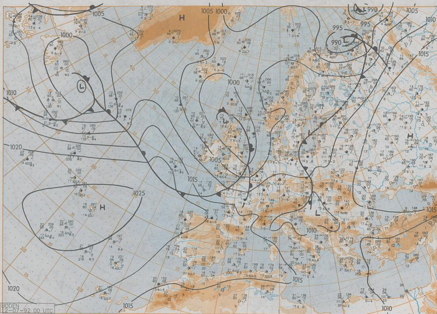
BODEN 12-07-92 00 UTC Stereogr.-proj. 1:30 000 000 60°N
