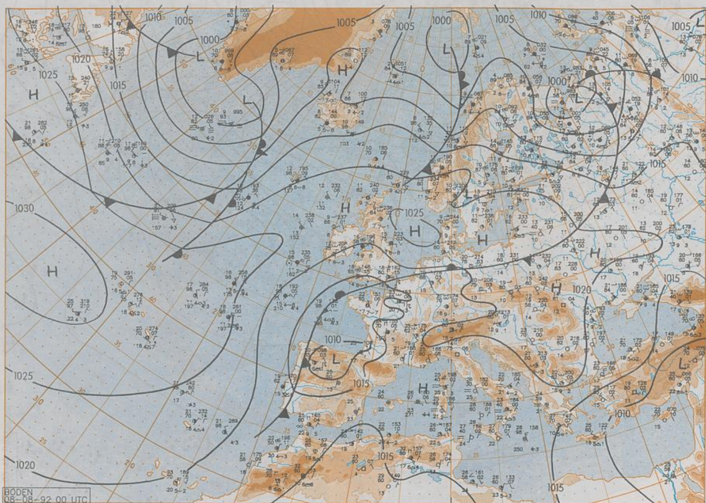
BODEN 08-08-92 00 UTC Stereogr. proj. 1:30 000 000 60°N
