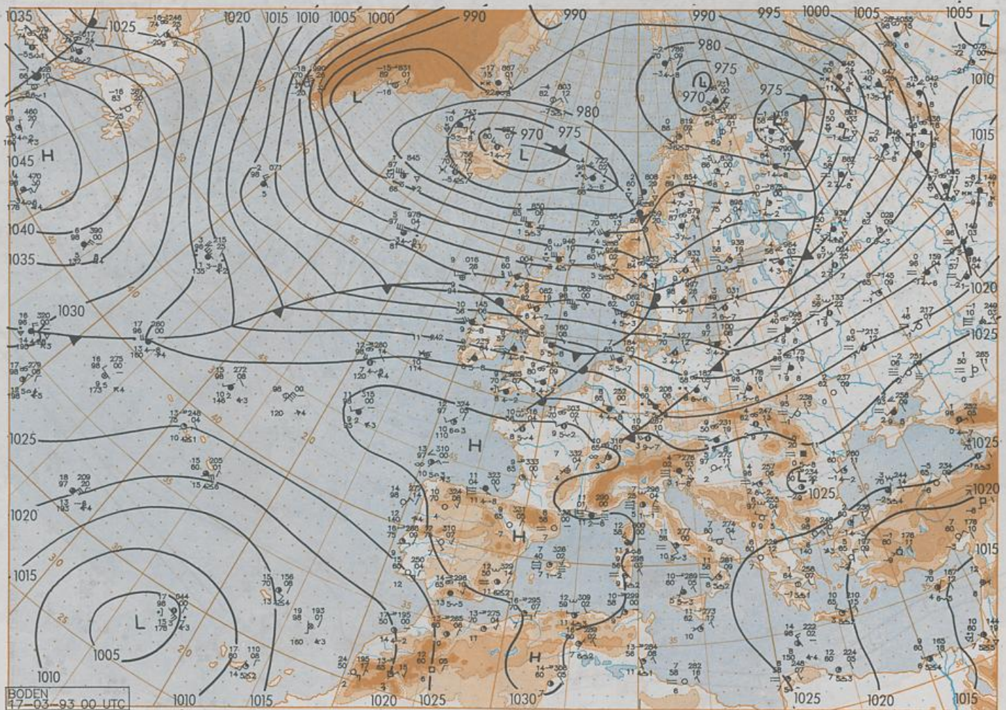
BODEN 17-03-93 00 UTC Stereogr. proj. 1:30 000 000 60°N
