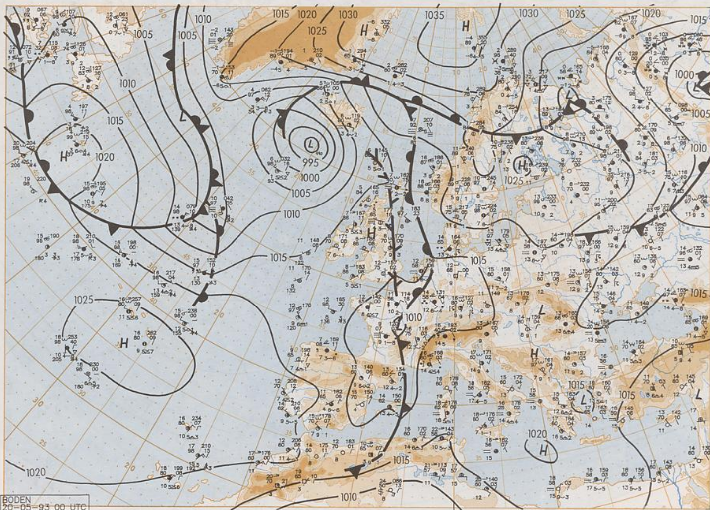
BODEN 20-05-93 00 UTC Stereogr. proj., 1:30 000 000 60°N
