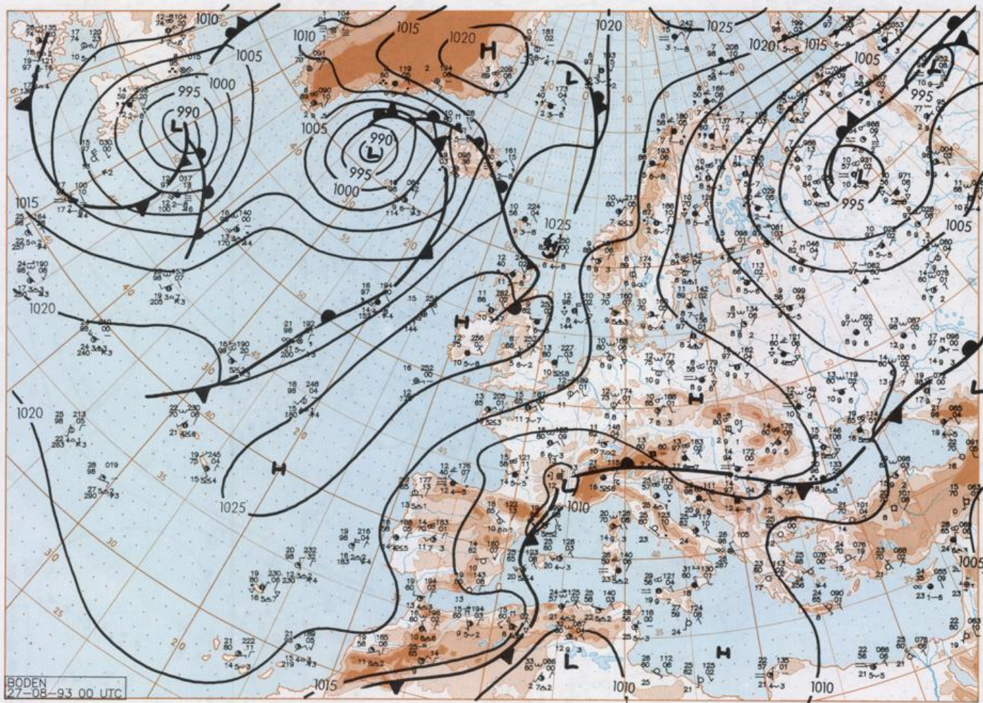
BODEN 27-08-93 00 UTC Steogr. proj. 1:30 000 000 60°N
