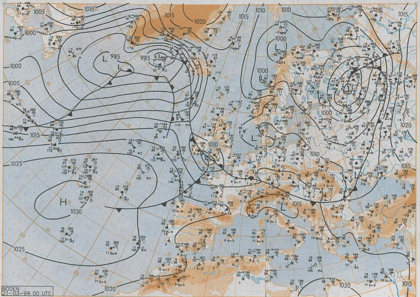
BODEN 21-03-94 00 UTC Stereogr. proj. 1:30 000 000 60°N
