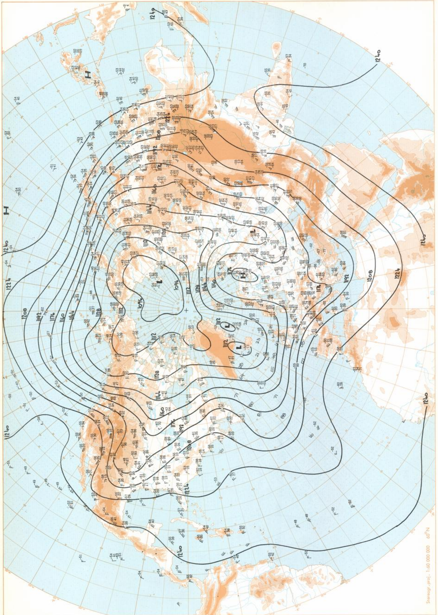
200 mbar 00 GMT
