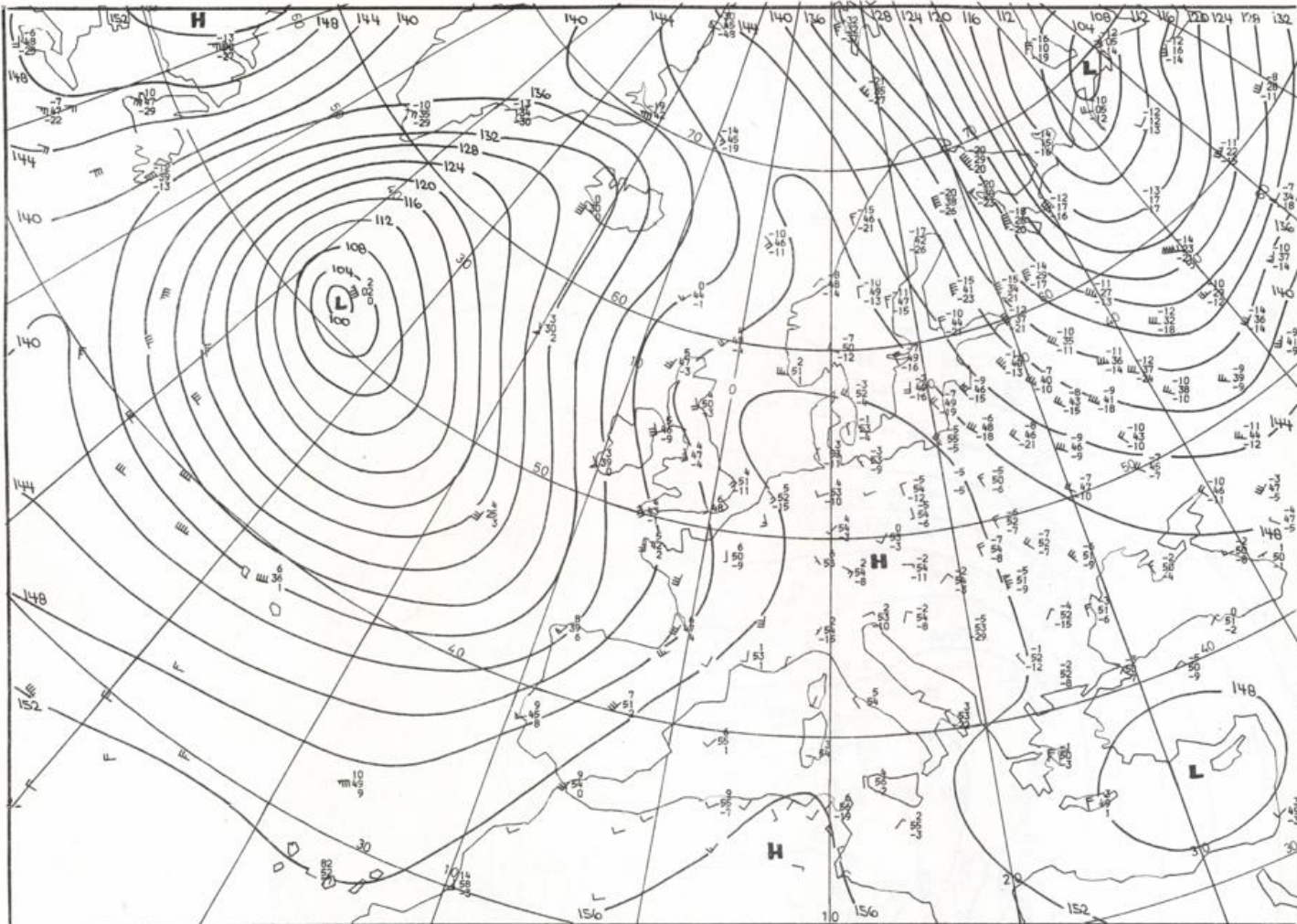
850 mbar 00 GMT
