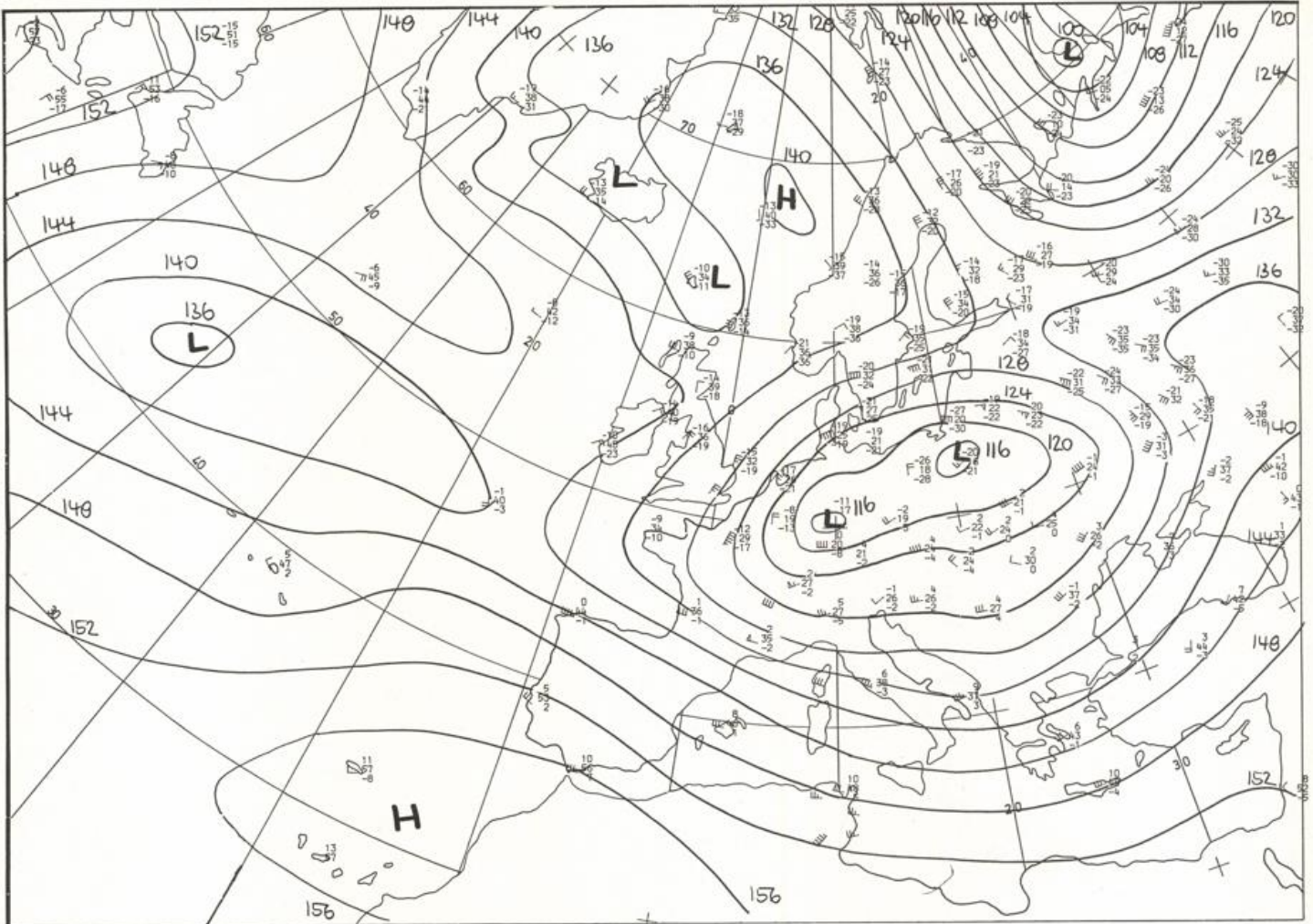
850 mbar 00 GMT
