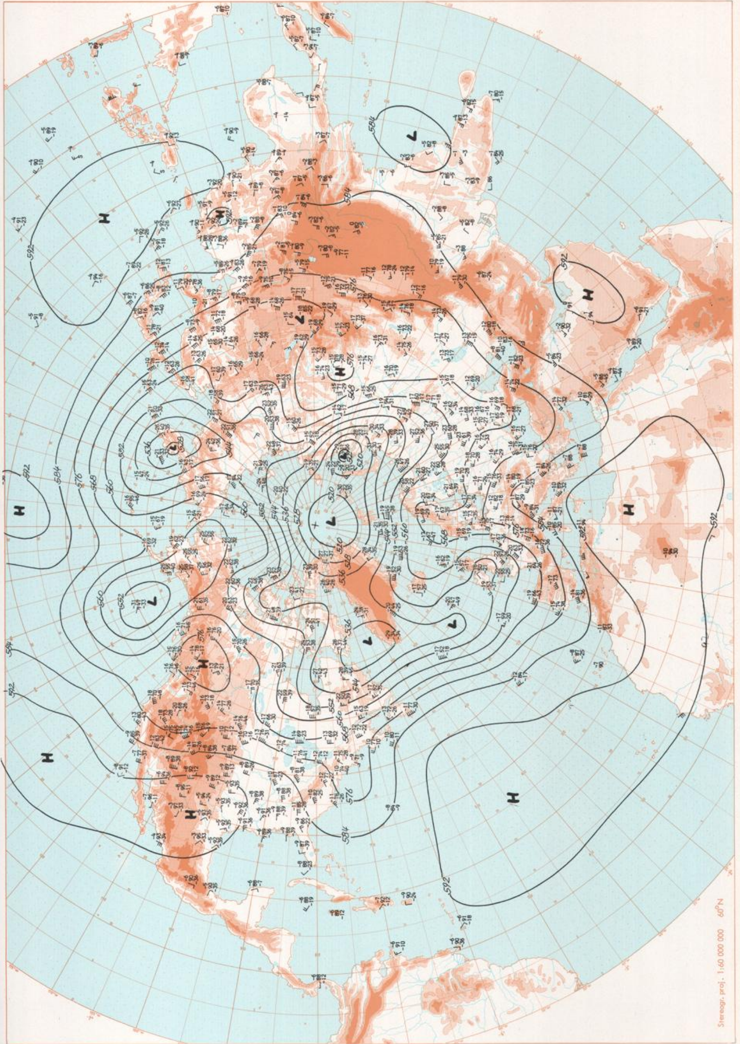
500 mb 00 GMT
