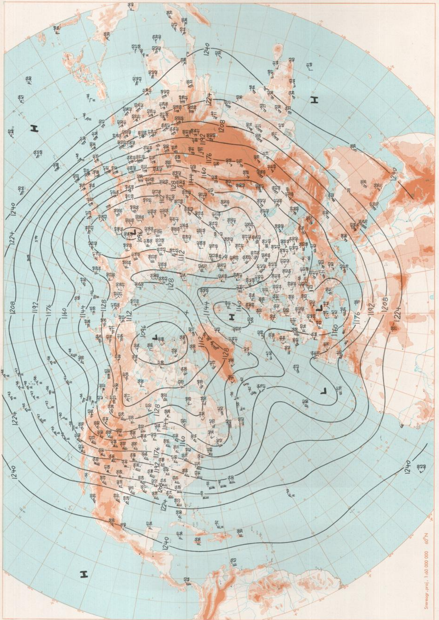
200 mbar. 00 GMT
