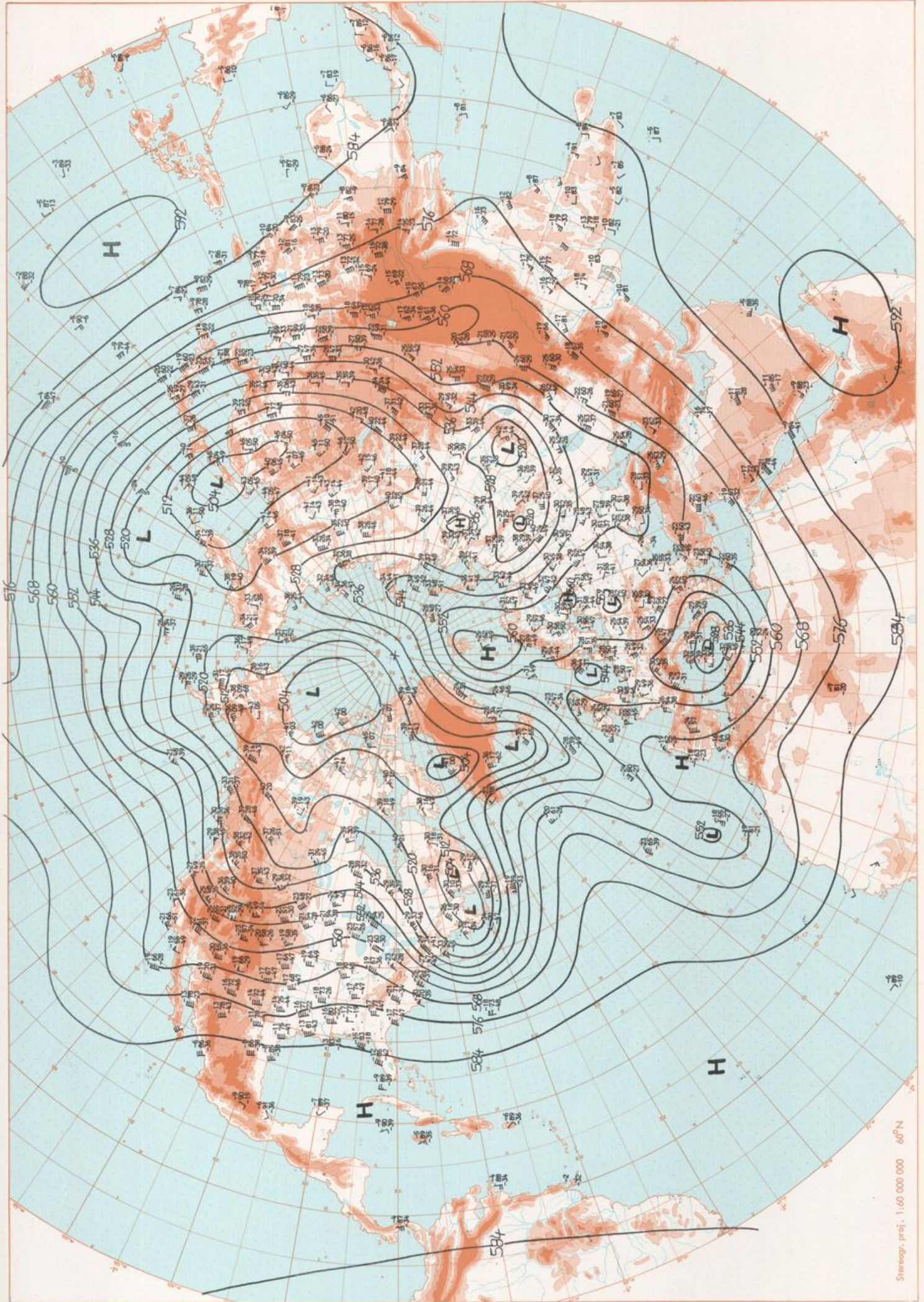
500 mbar ○ GMT
