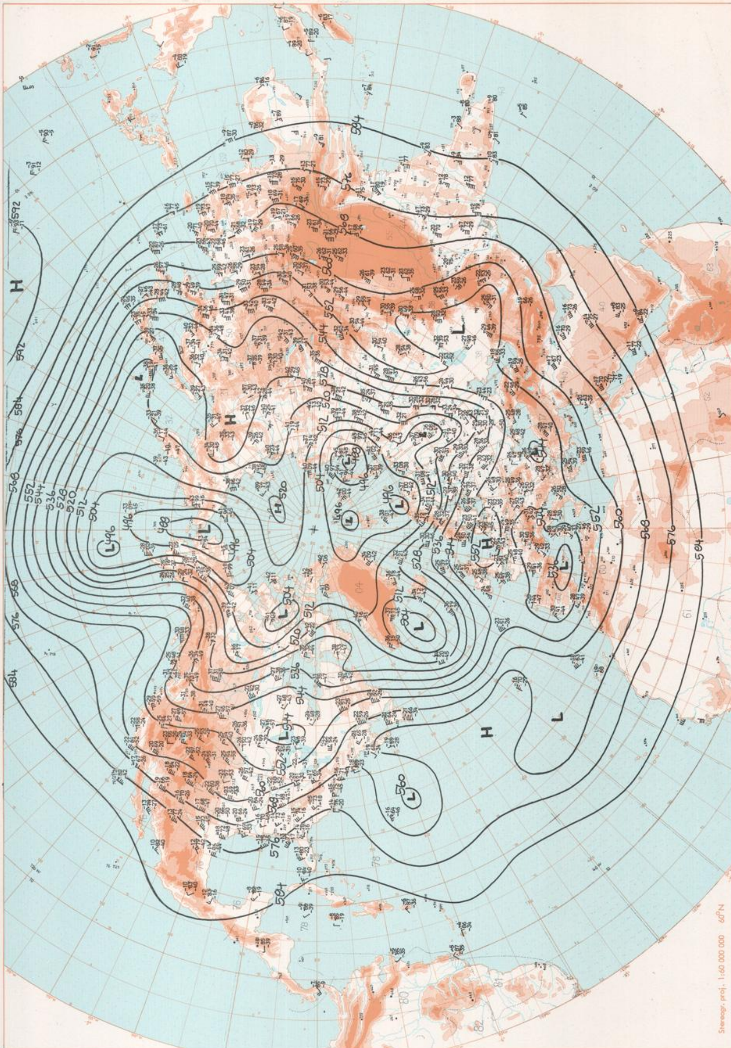
500 mbar 00 GMT
