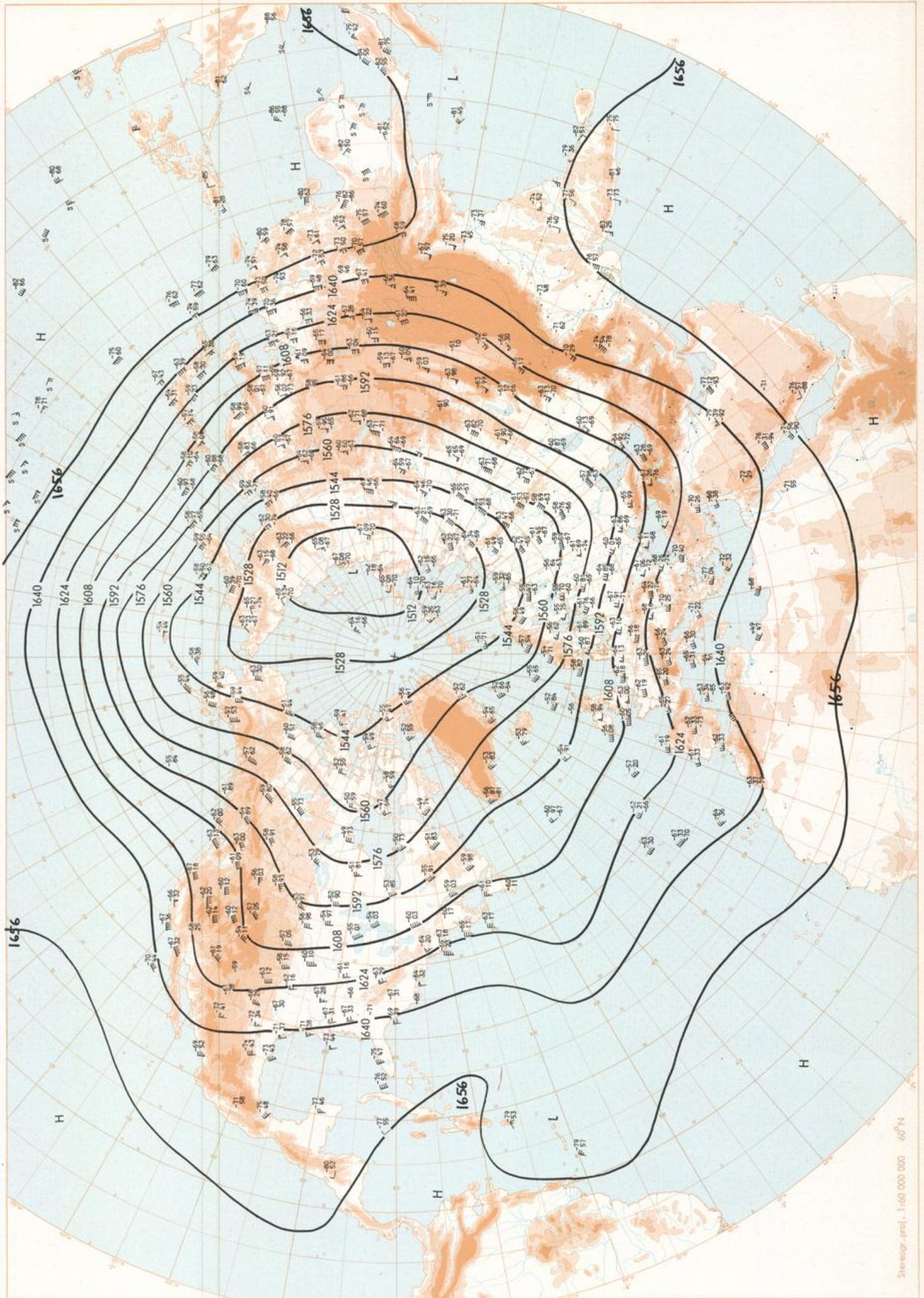
100 mbar 00 GMT
