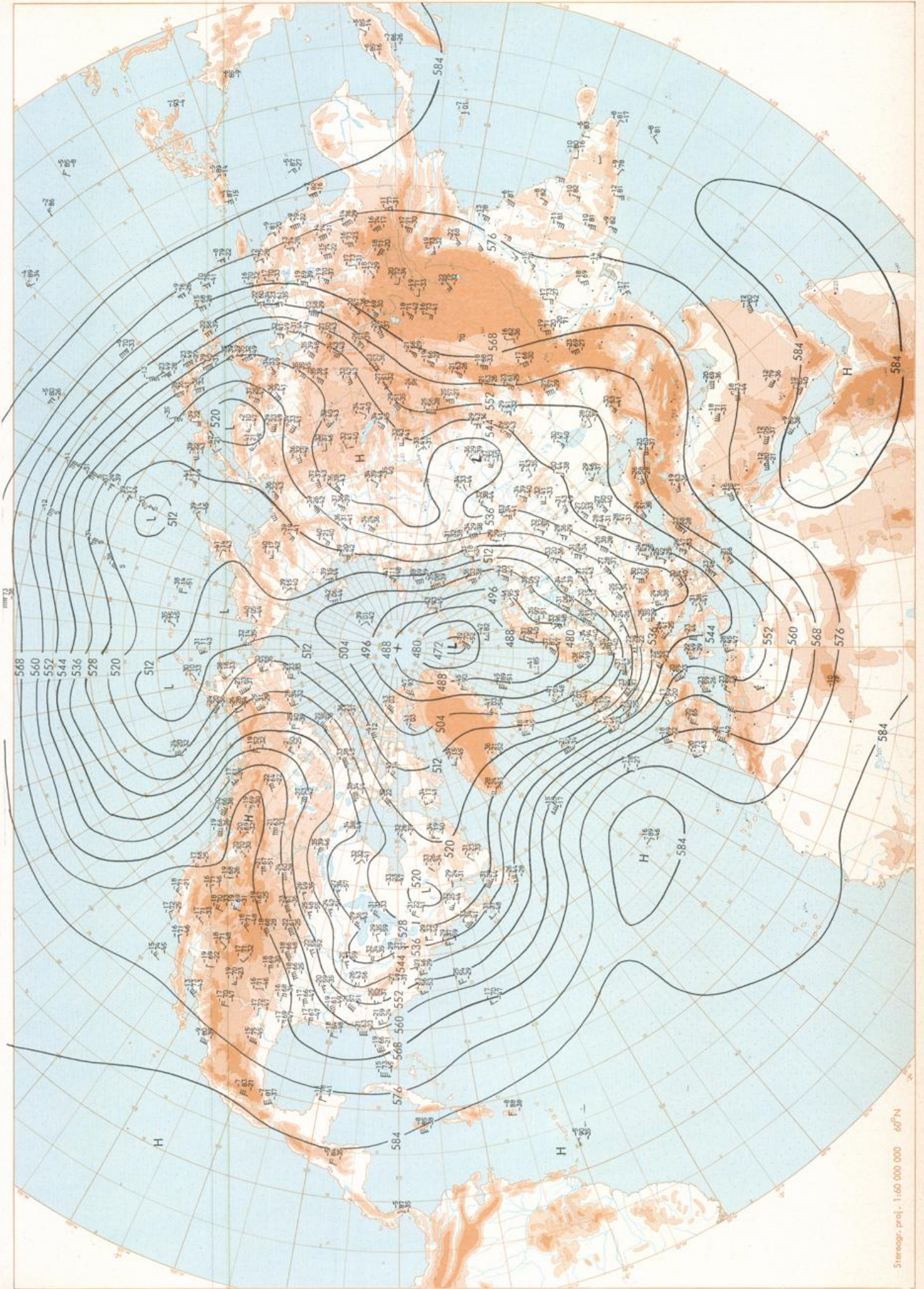
500 mbar 00 GMT
