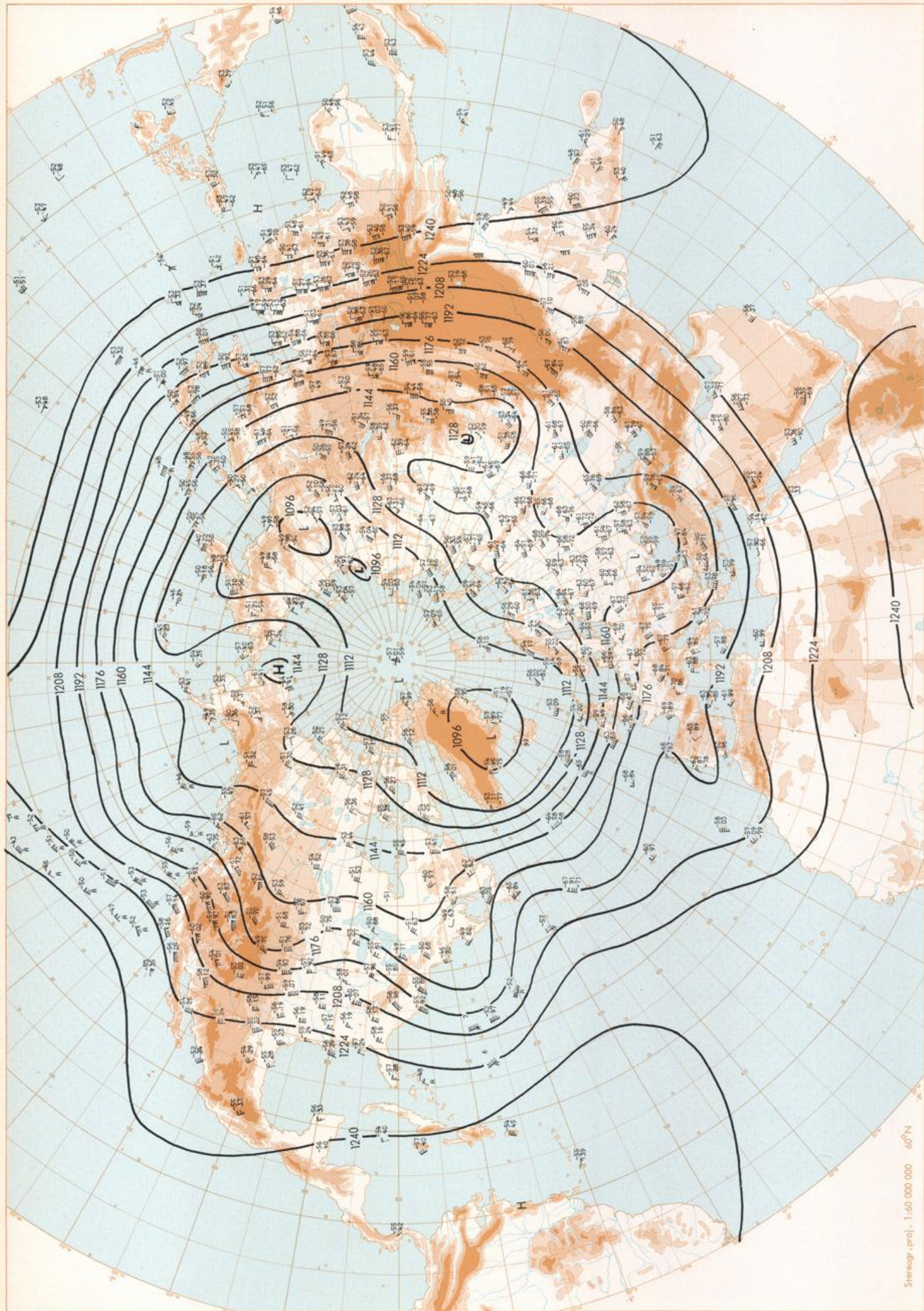
200 mbar 00 GMT
