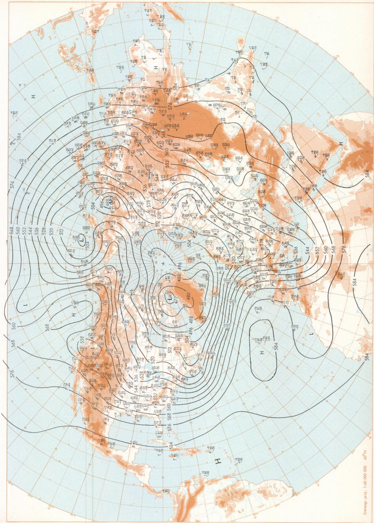
500 mbar 00 GMT
