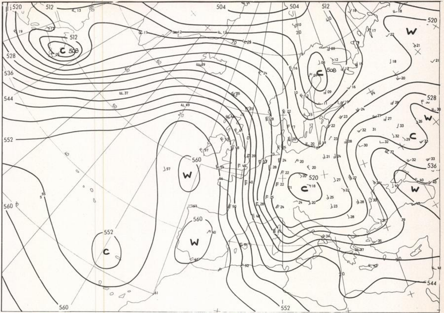
Stereogr.proj. 1:30 000 000 60°N
