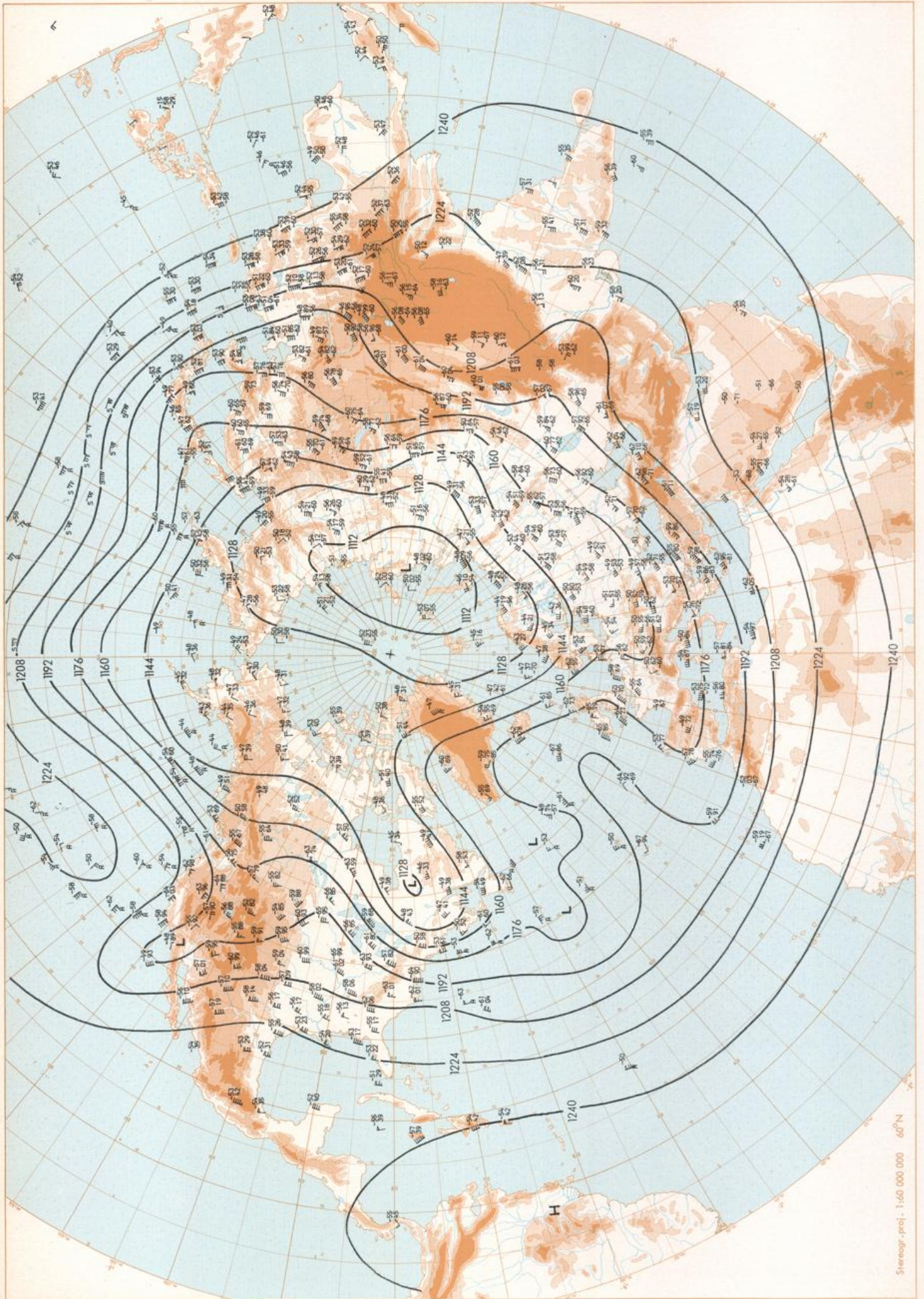
200 mbar ○ GMT
