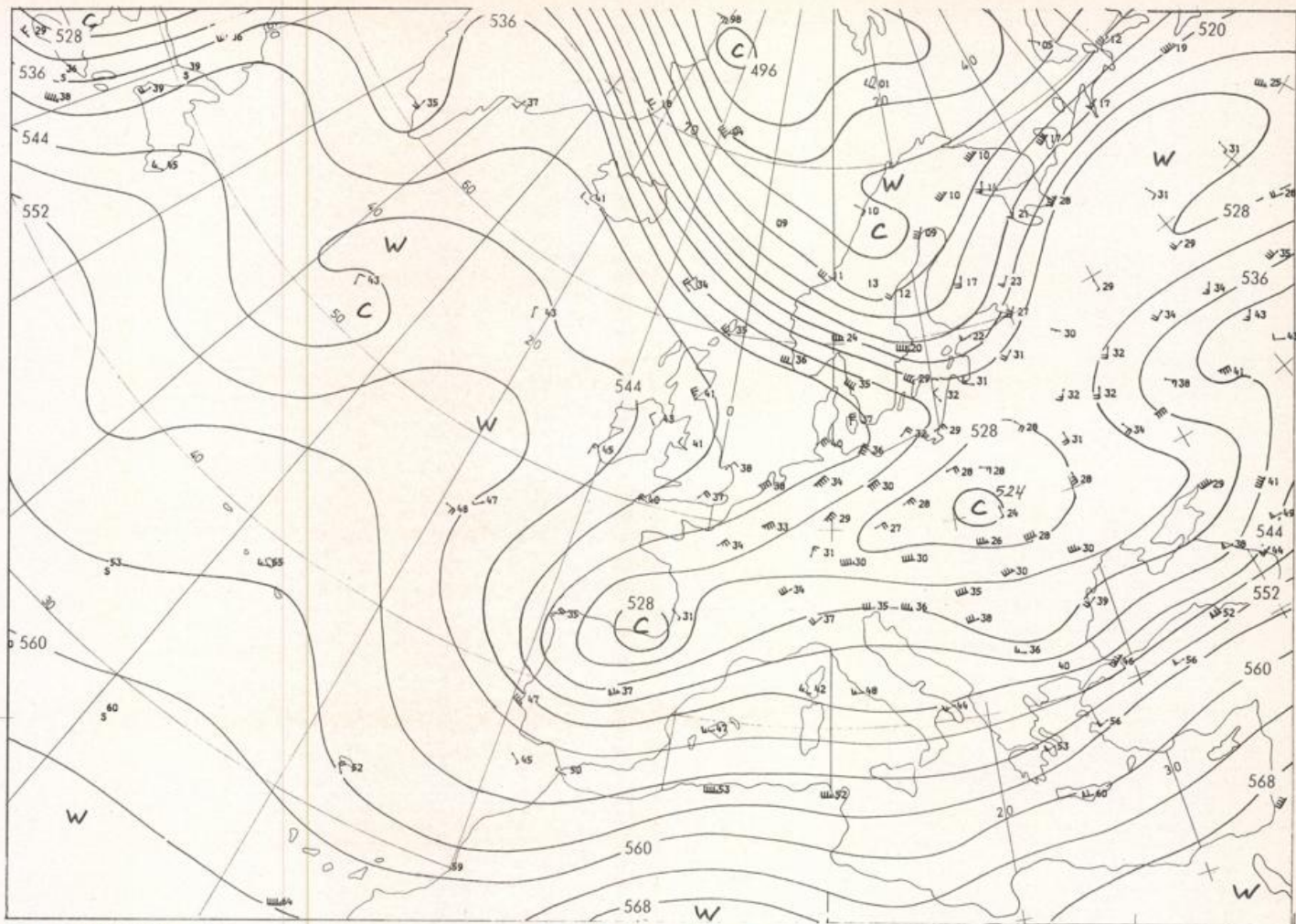
Stereogr.proj. 1:30 000 000 60°N
