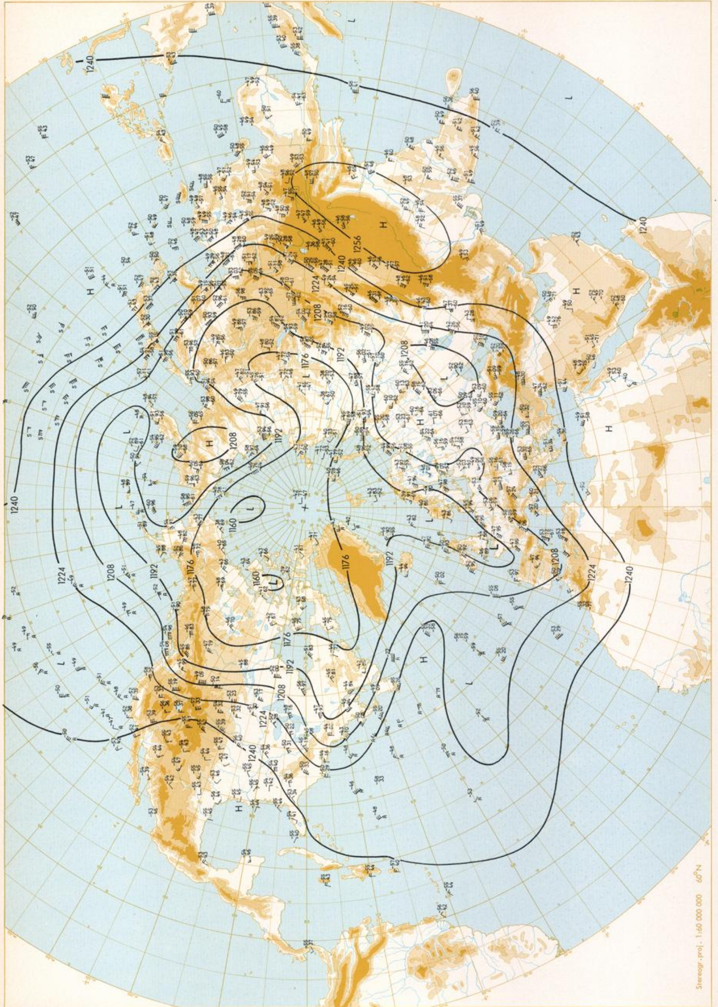
200 mbar 00 GMT
