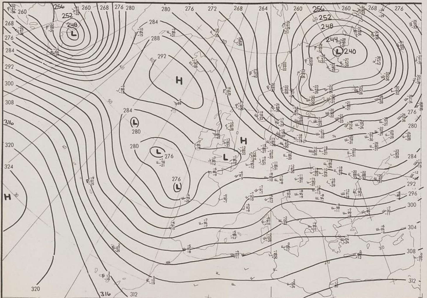
700 mbar 00 GMT
