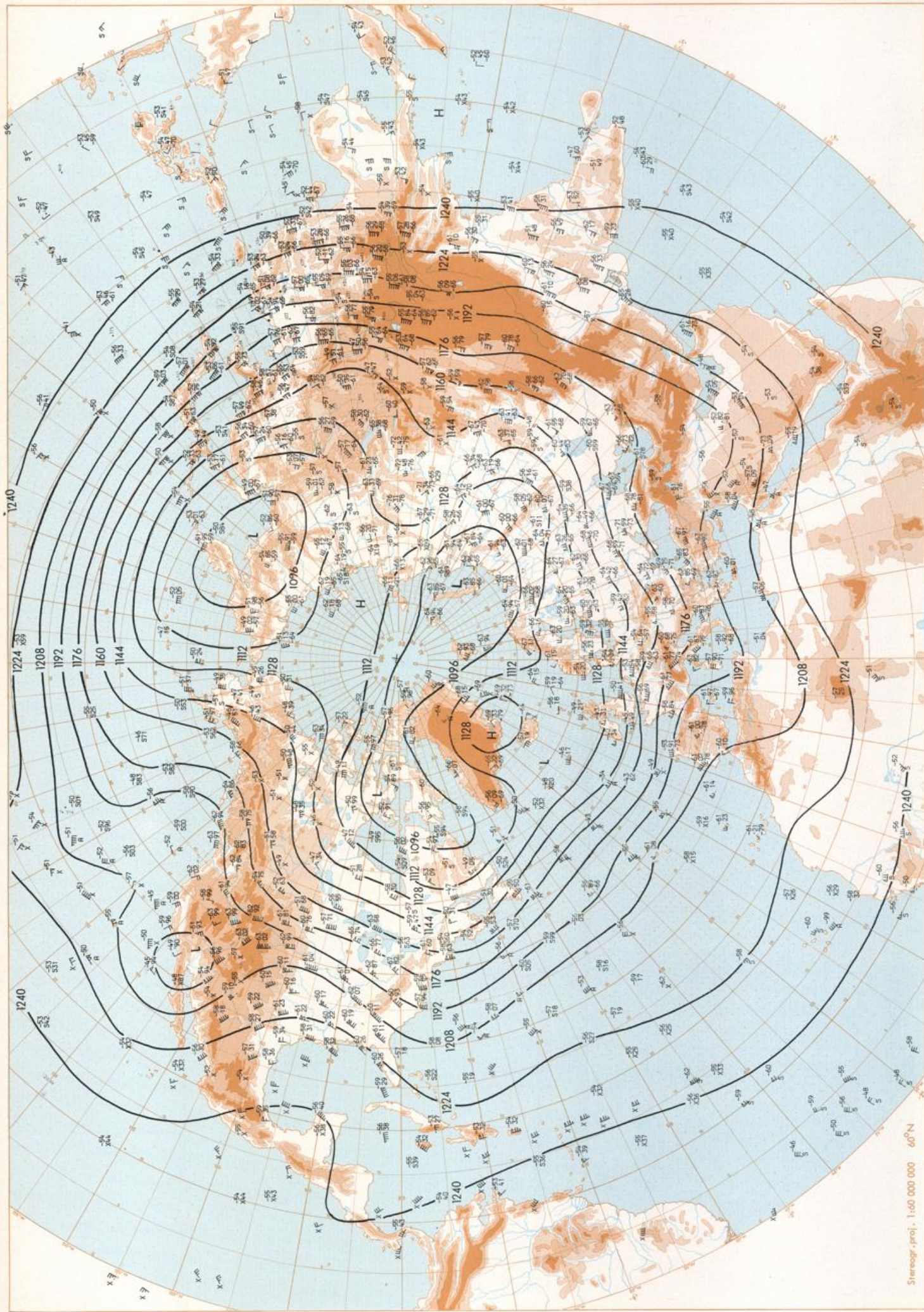
200 mbar QQ GMT
