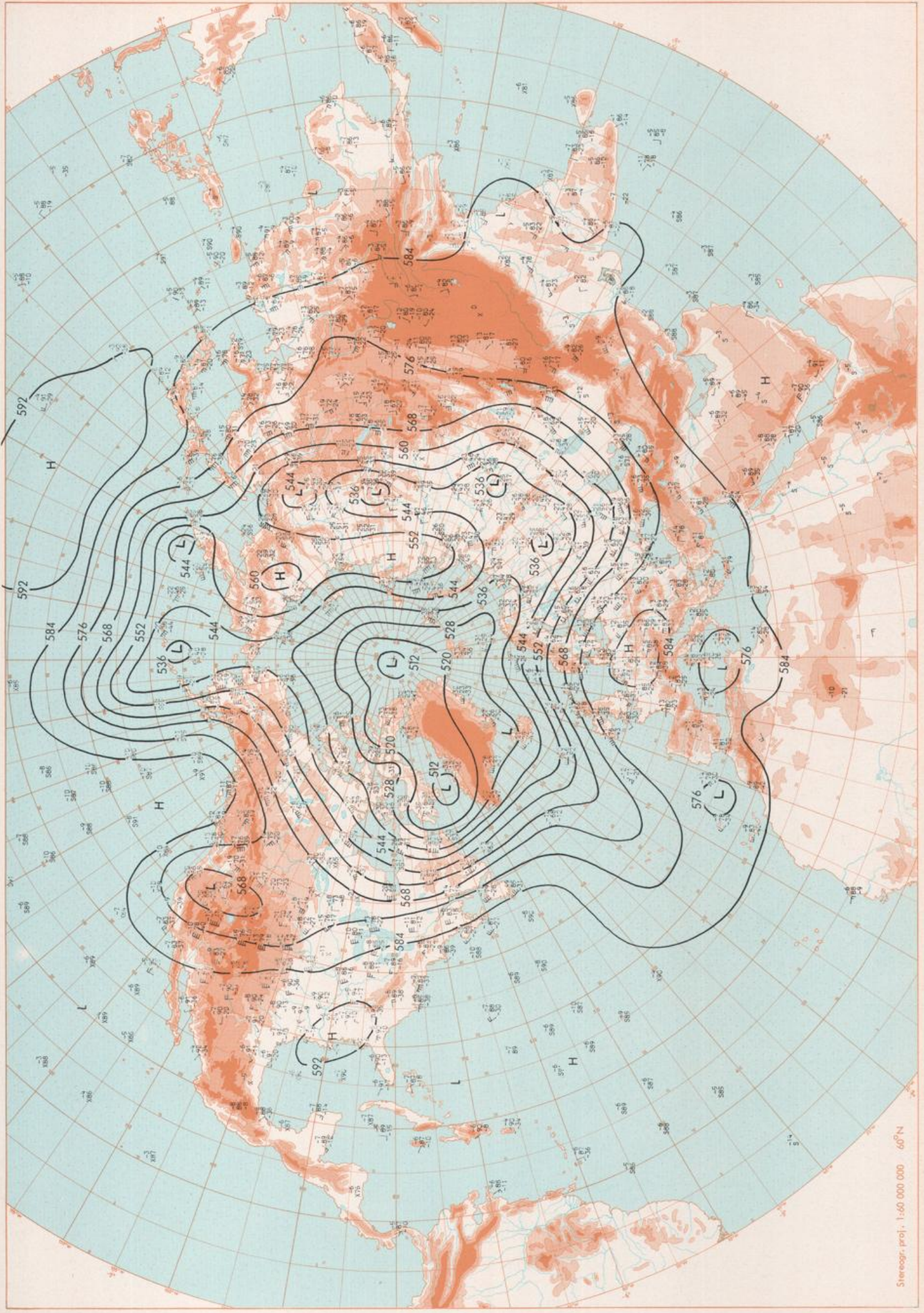
500 mbar 00 GMT
