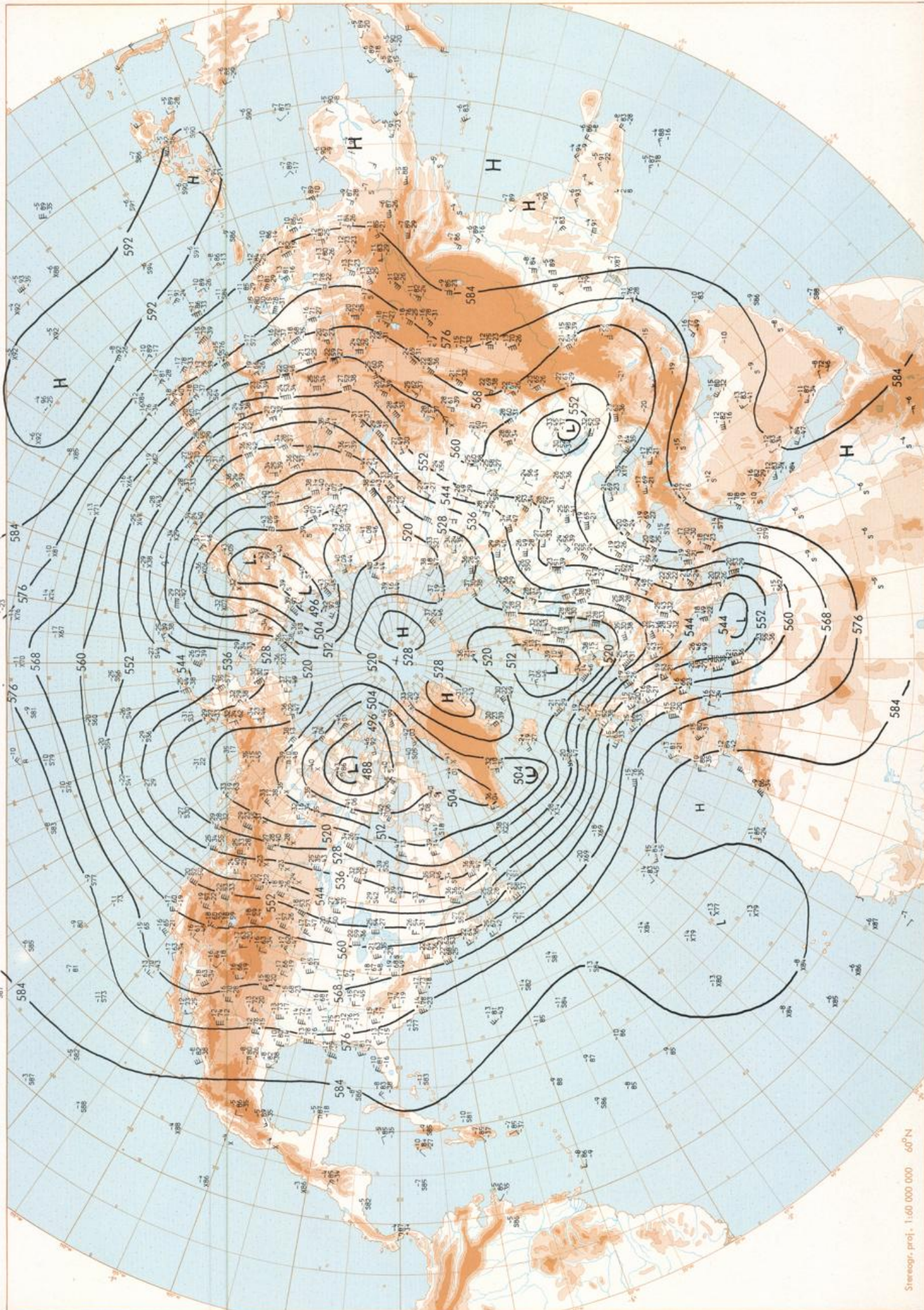
500 mbar 00 GMT
