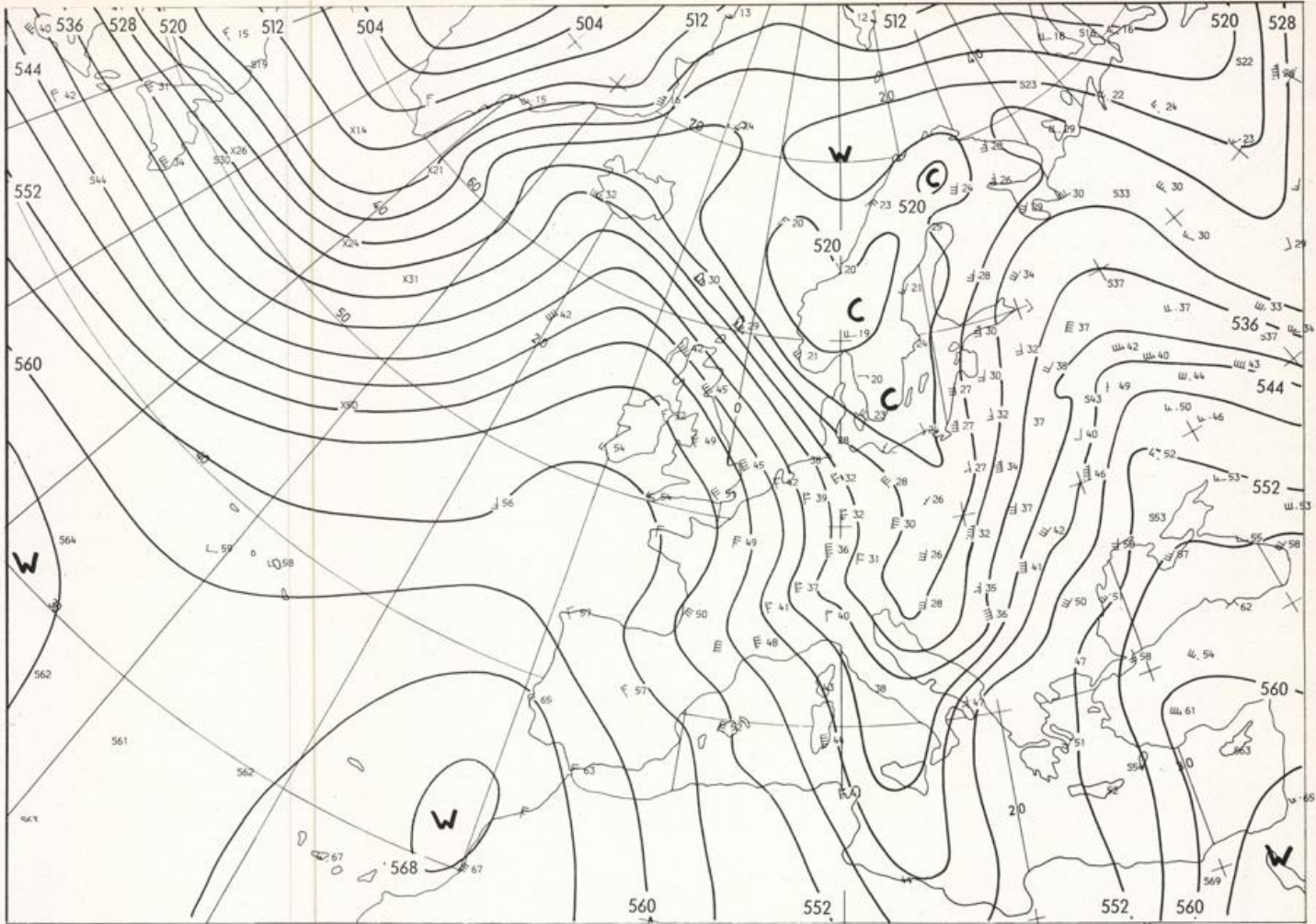
Stereogr.-proj. 1:30 000 000 60°N
