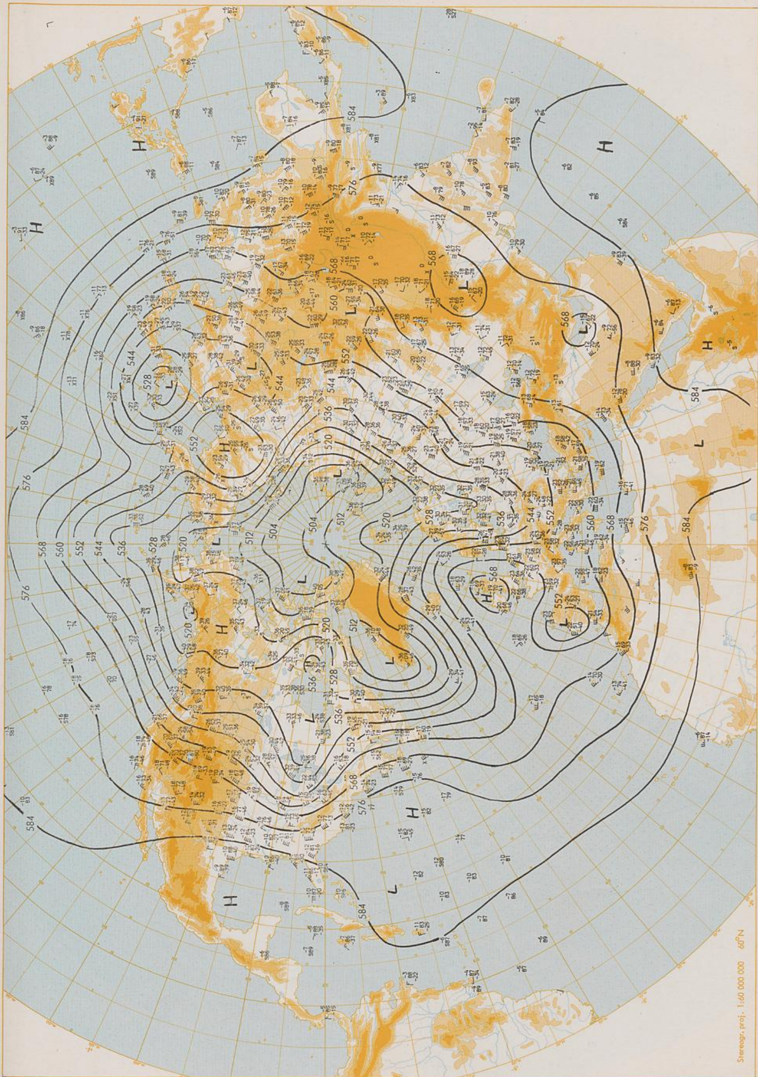
500 mbar 00 GMT
