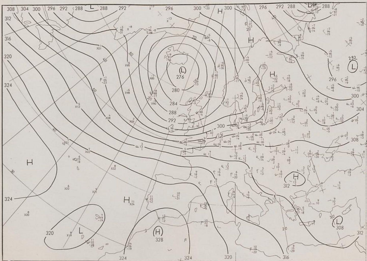
700 mbar 00 GMT
