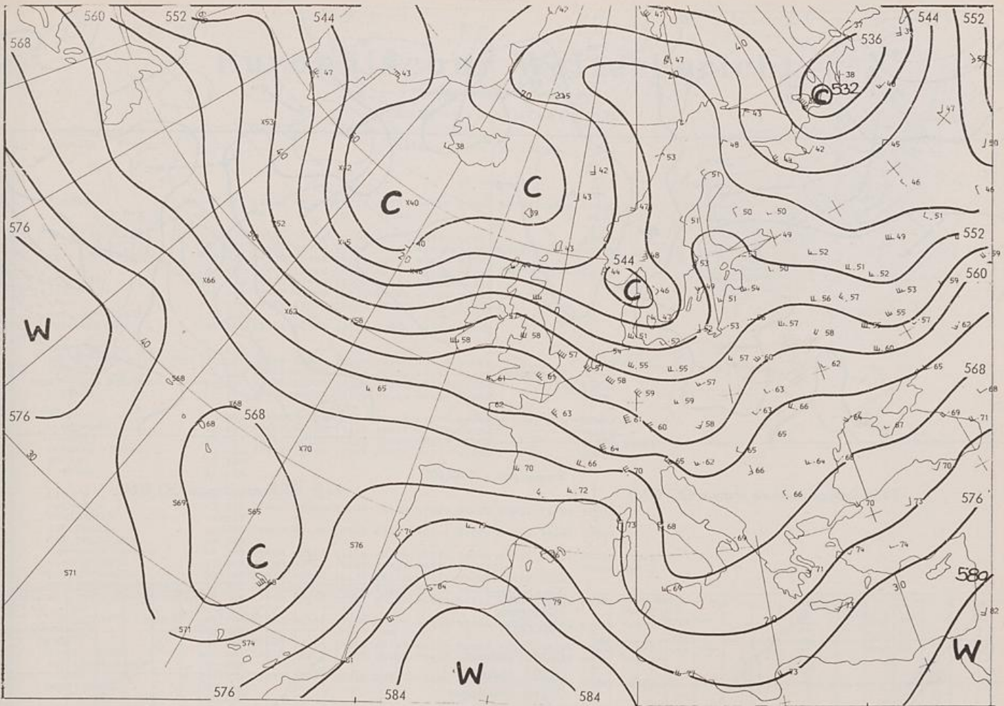
500/1000 mbar 00 GMT
