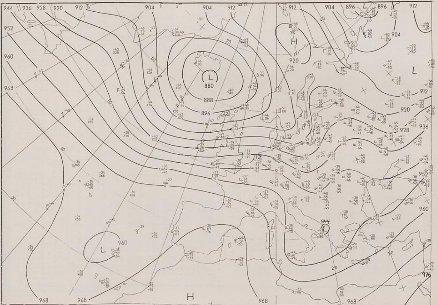
300 mbar 00 GMT
