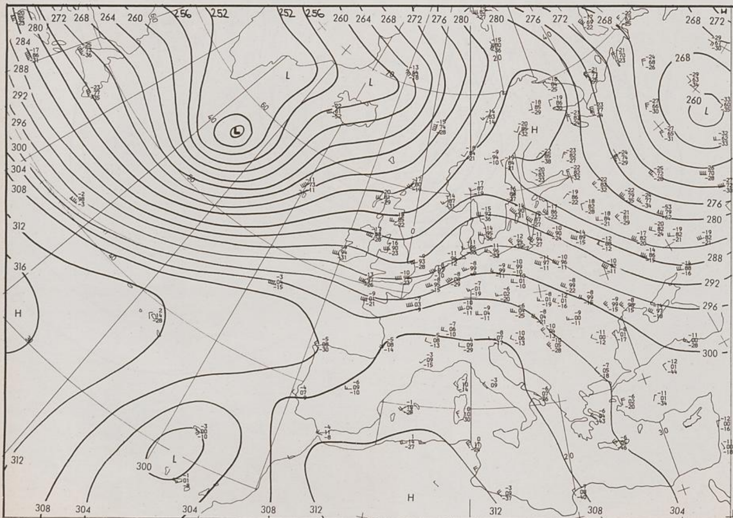
700 mbar 00 GMT
