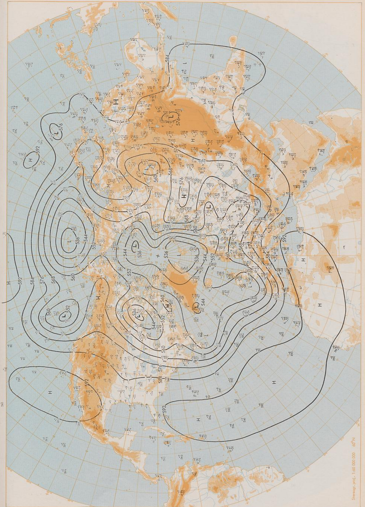
500 mbar 00 GMT
