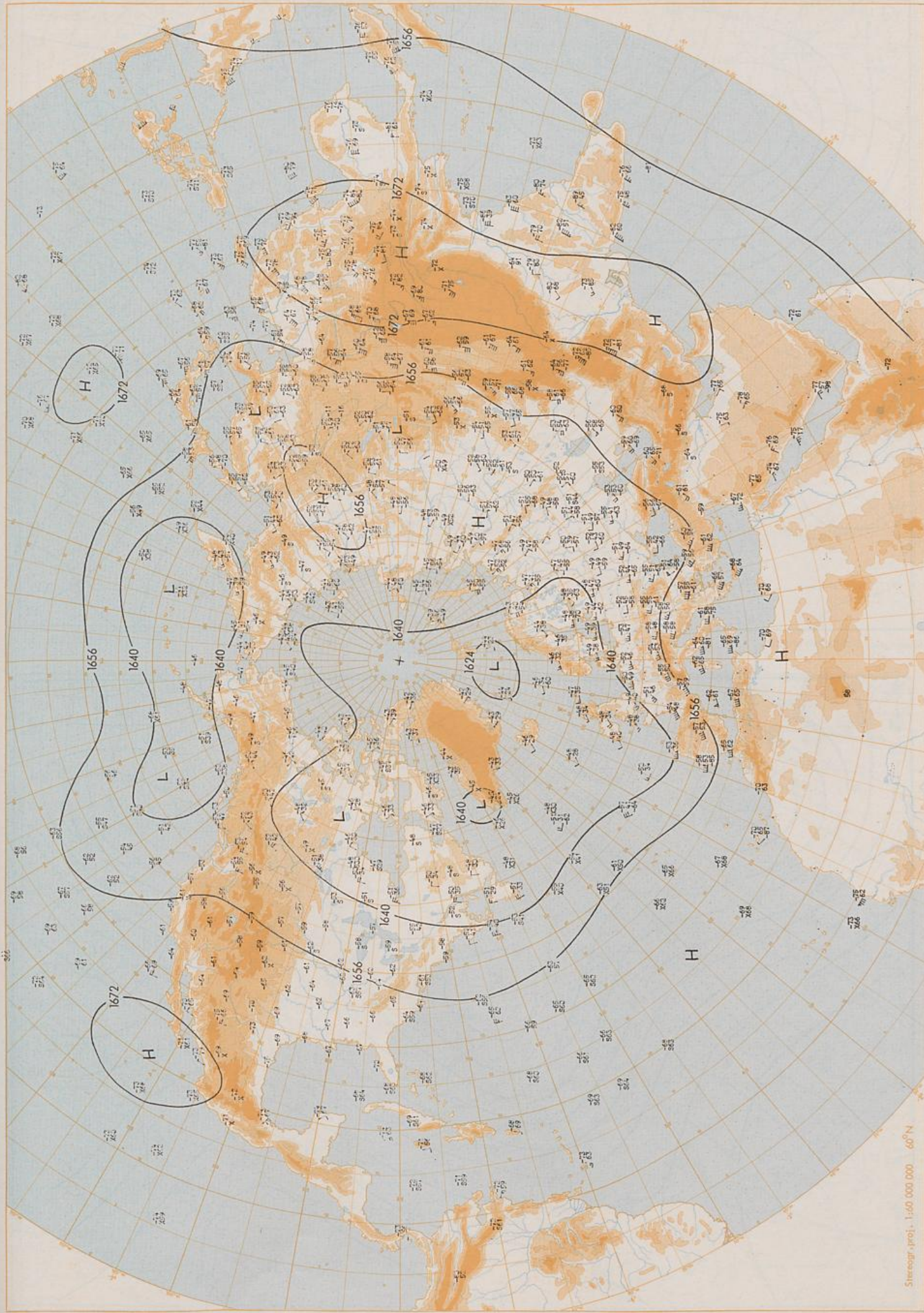
100 mbar 00 GMT
