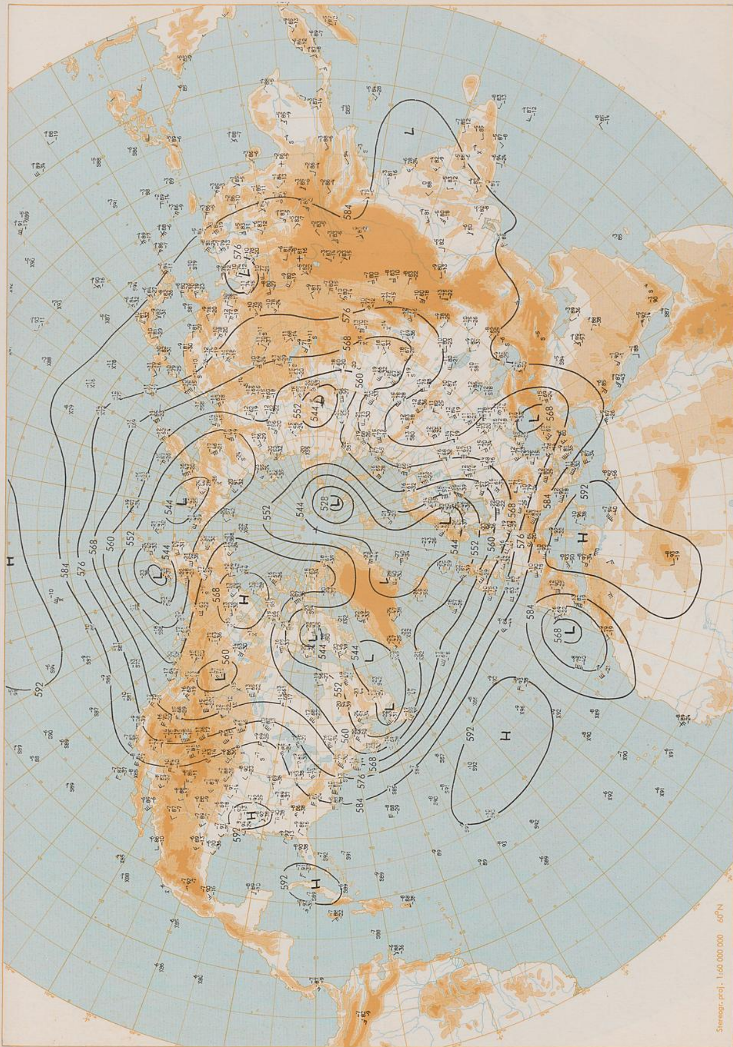
500 mbar 00 GMT
