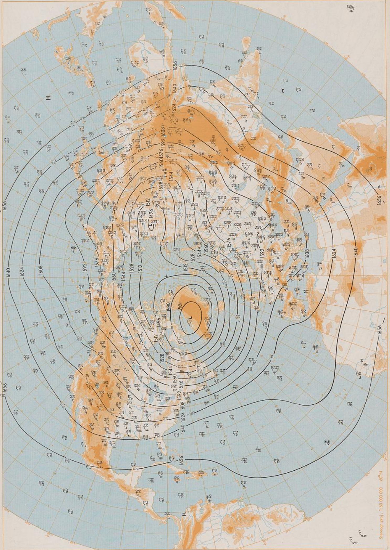
100 mbar 00 GMT
